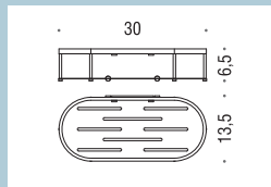
B9641 Angolare sganciabile per box doccia Removable single corner basket for shower
